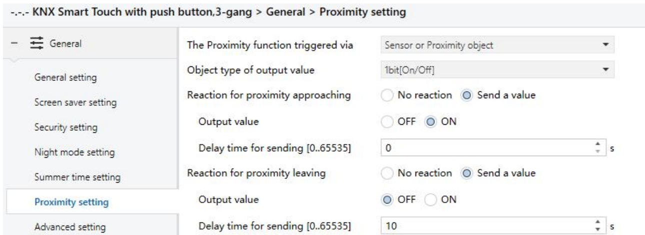
图 5.1.6 “Proximity setting” 参数设置界面
