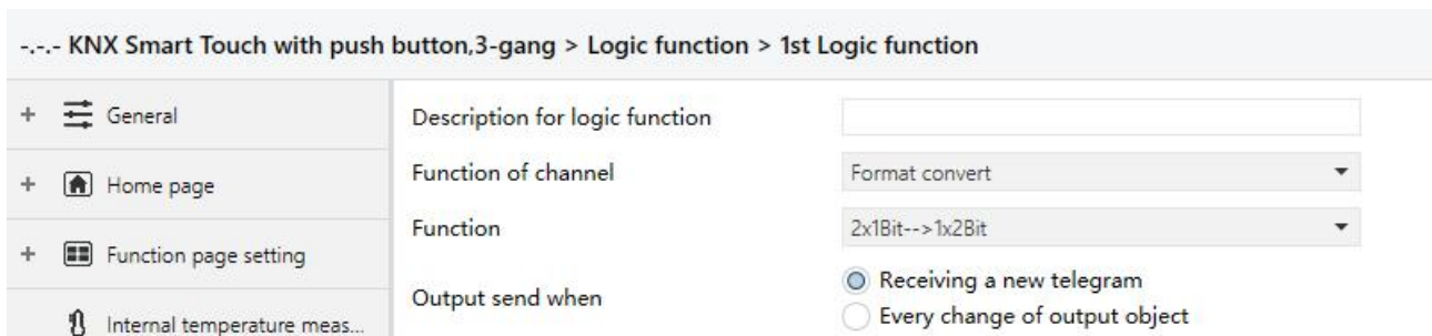
图 5.8.4 “Format convert” 功能参数
