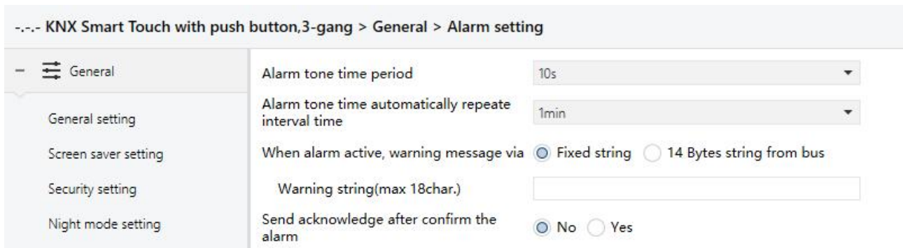
图 5.1.8 “Alarm setting” 参数设置界面
