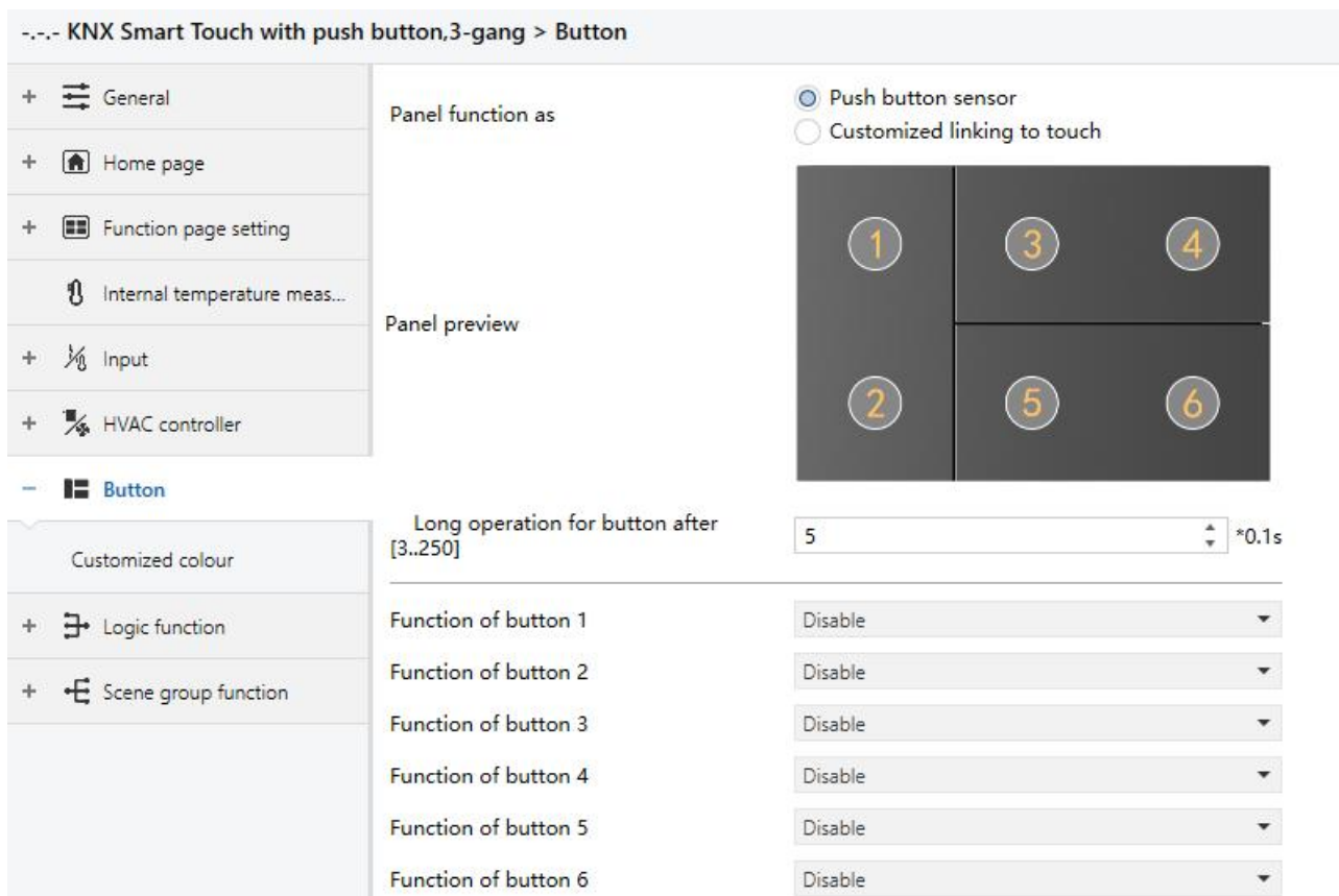
图 5.7.1 按键功能设置参数
