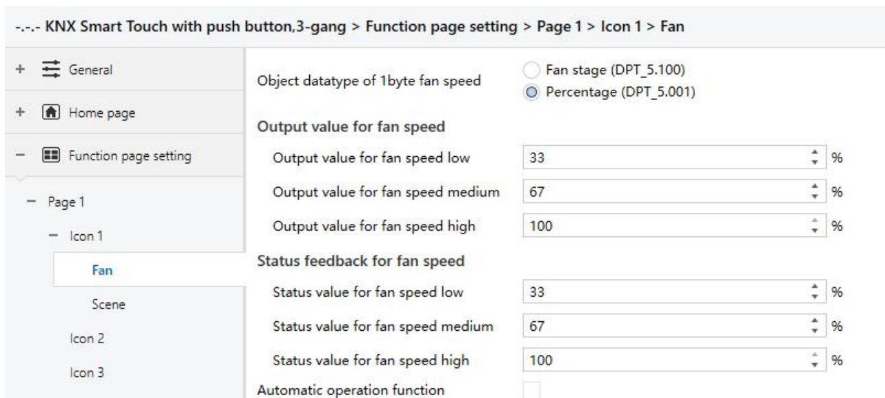
图 5.6.2.3(2) 温控-风速参数设置界面
