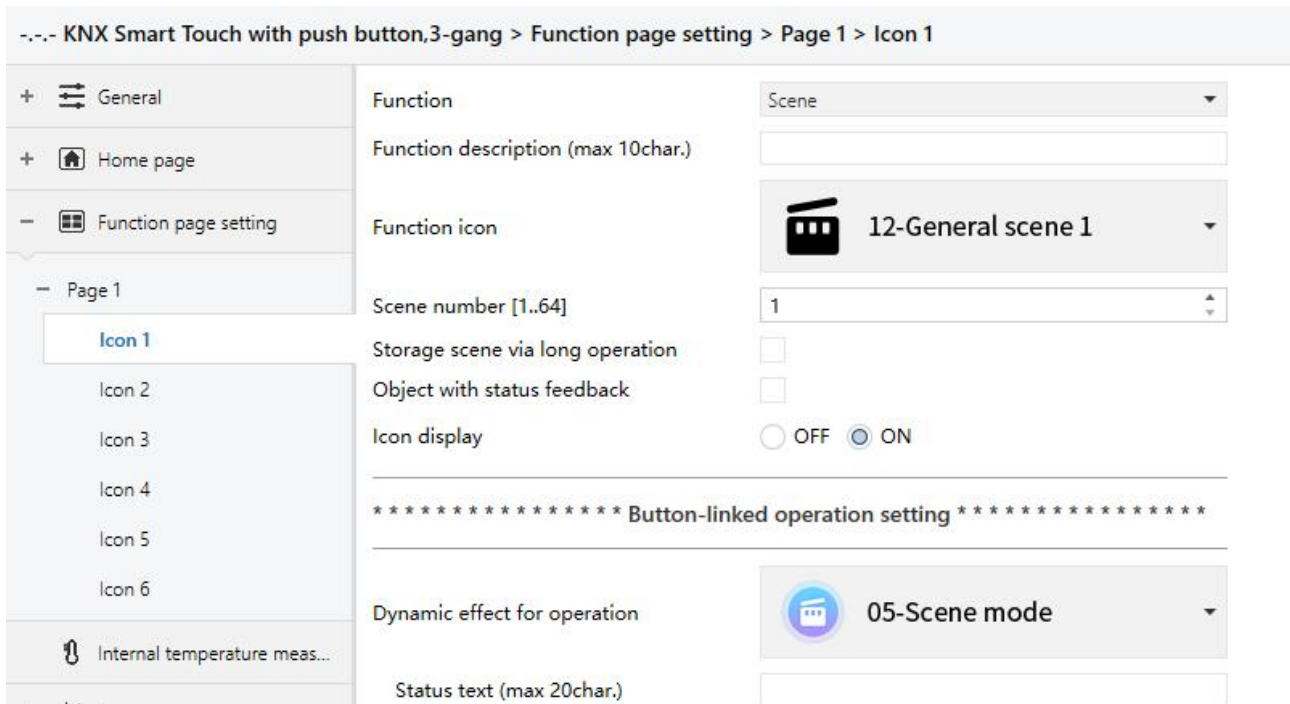
图 5.6.2.1 (7) 场景功能参数设置
