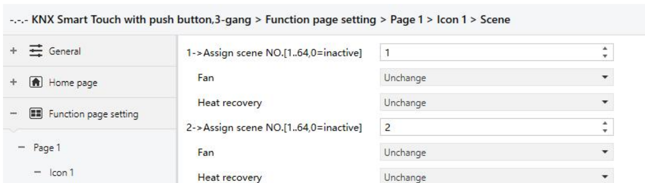
图 5.6.2.4(2) 新风-场景参数设置界面
