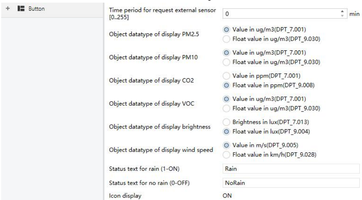
图 5.1.2 “Screen saver setting” 参数设置界面
