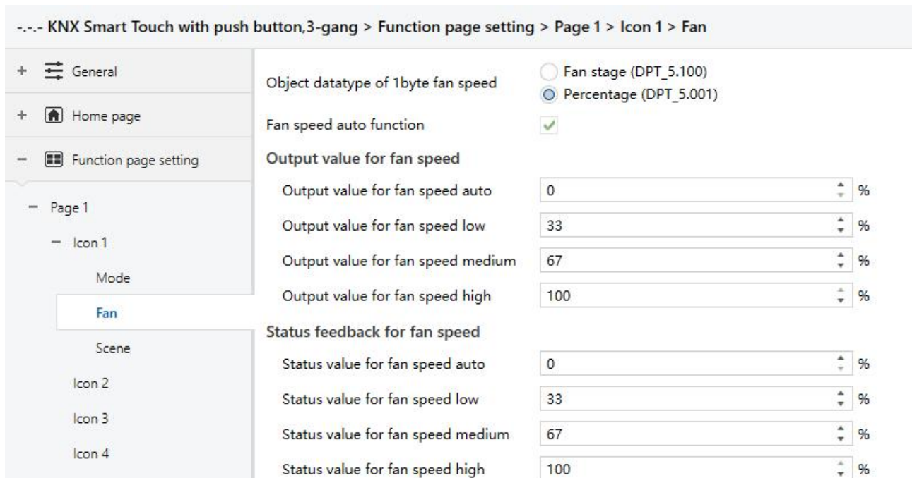
图 5.6.2.2(3) 空调-风速参数设置界面
