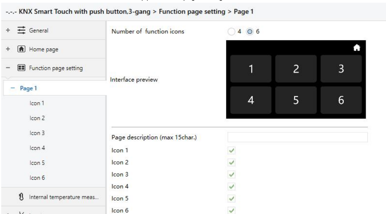
图 5.6.1(2) “Page x” 参数设置界面
