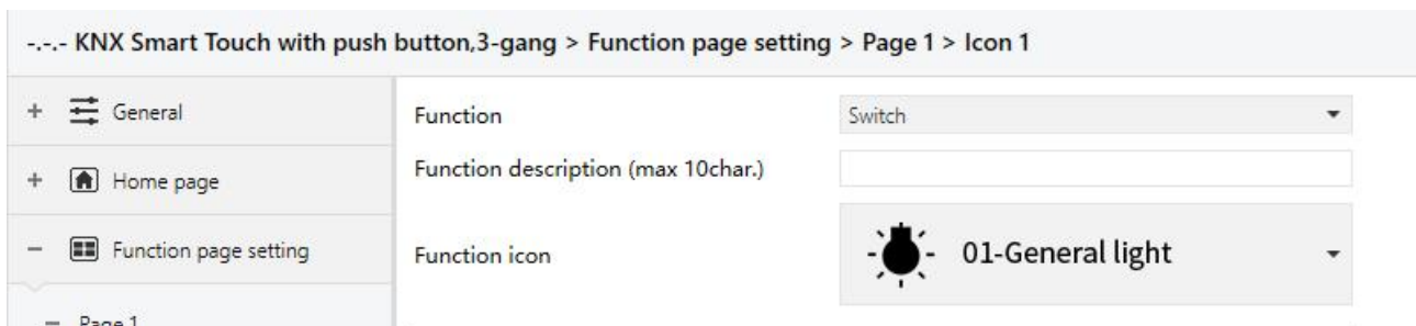
图 5.6.1 “Icon x” 参数设置界面
