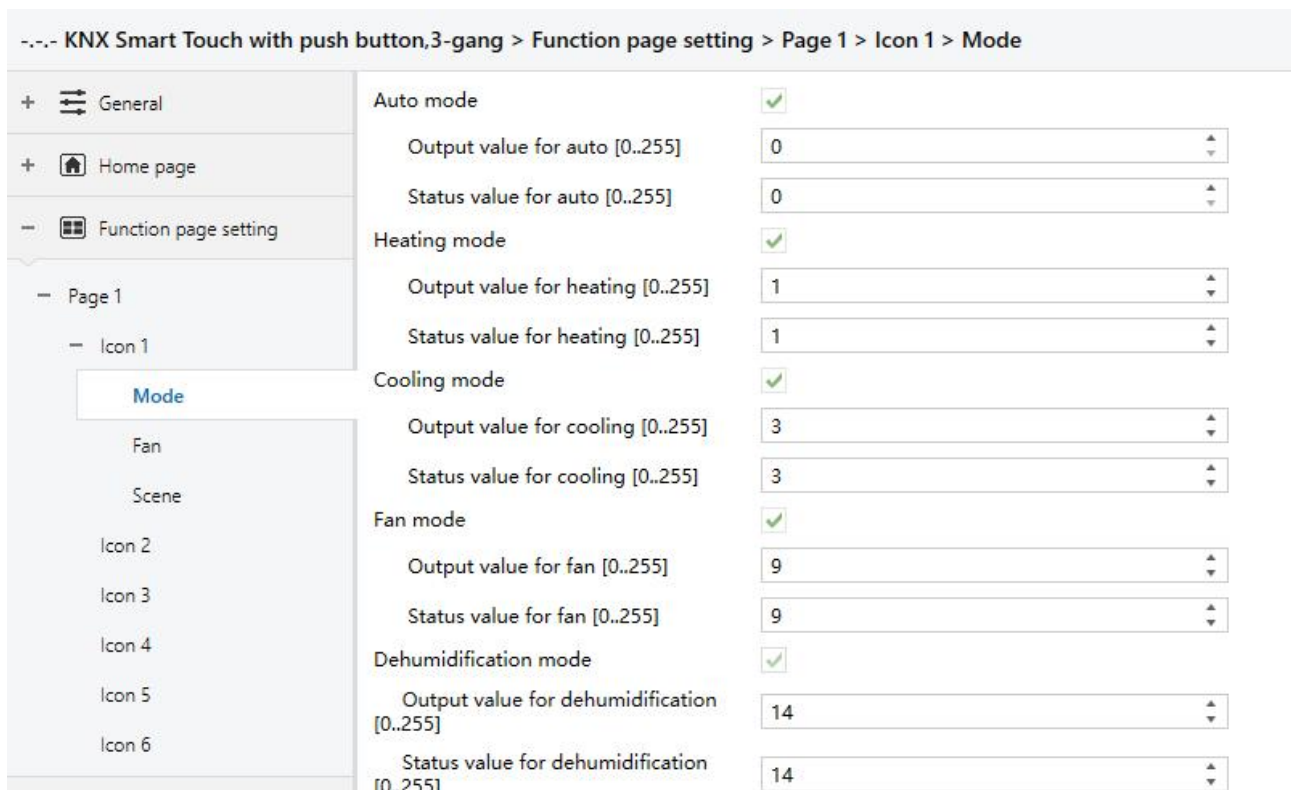
图 5.6.2.2(2) 空调-模式参数设置界面
