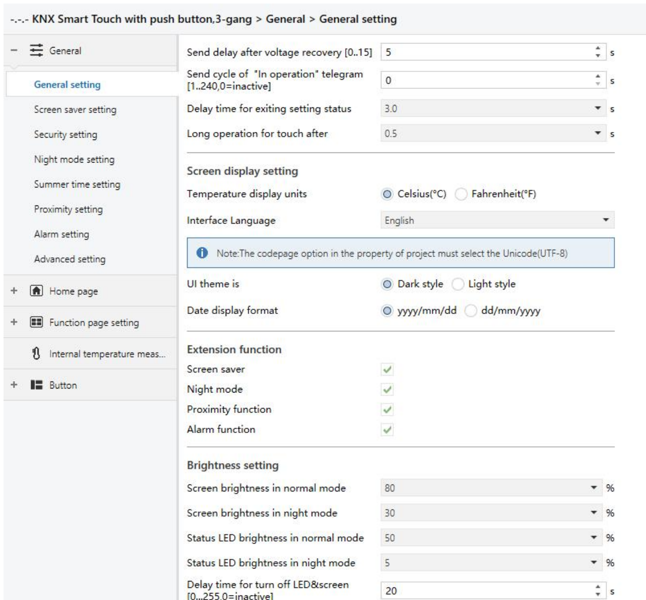
图 5.1.1 “General setting” 参数设置界面
