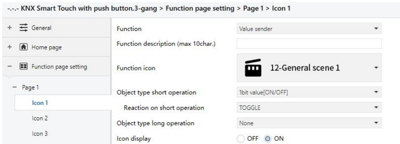
图 5.6.2.1 (6) 值发送功能参数设置
