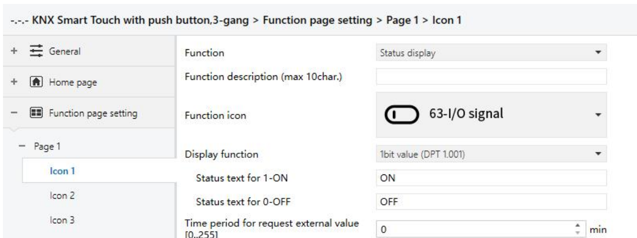
图 5.6.2.1(8) 状态指示功能参数设置
