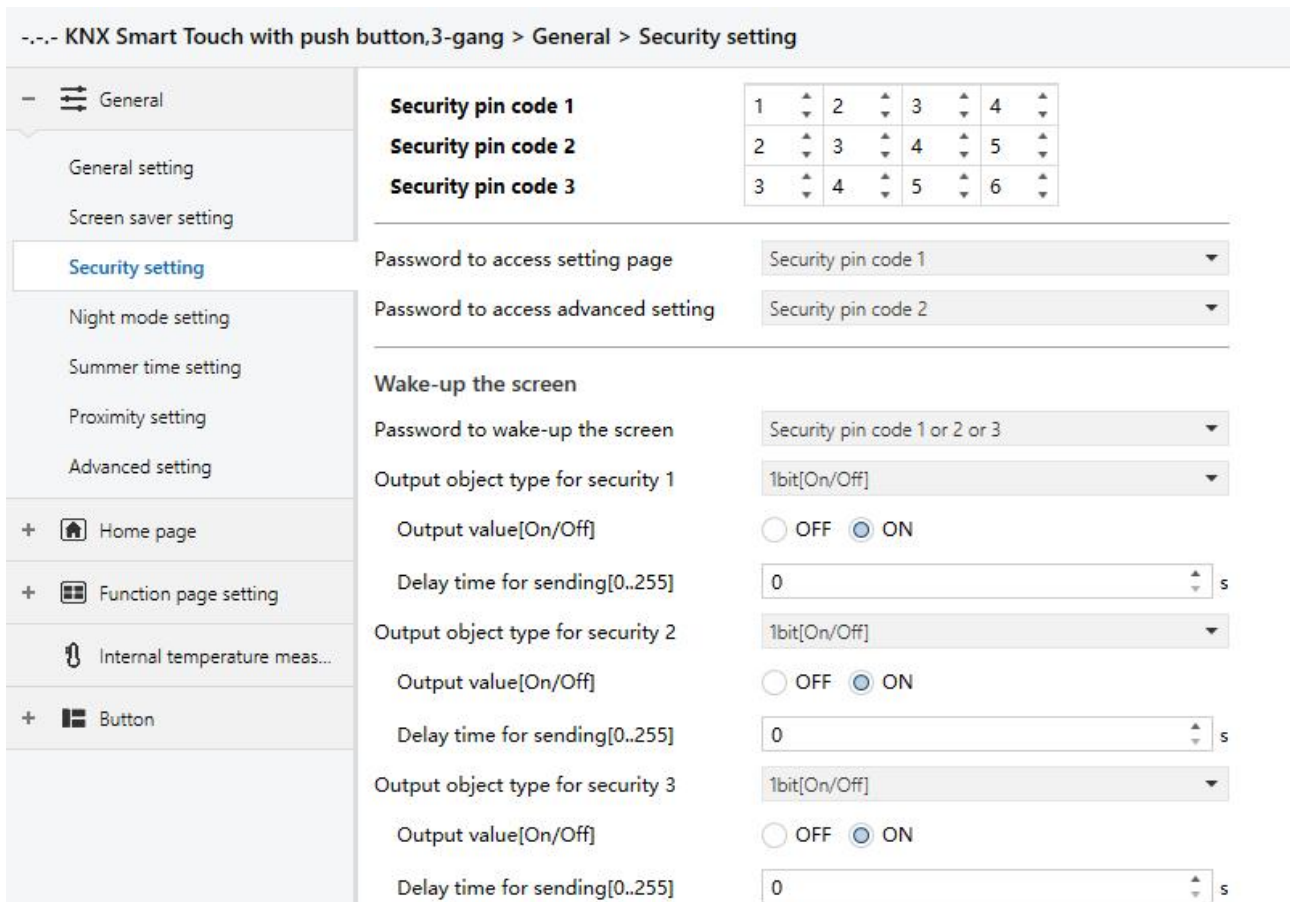
图 5.1.3 “Security setting” 参数设置界面
