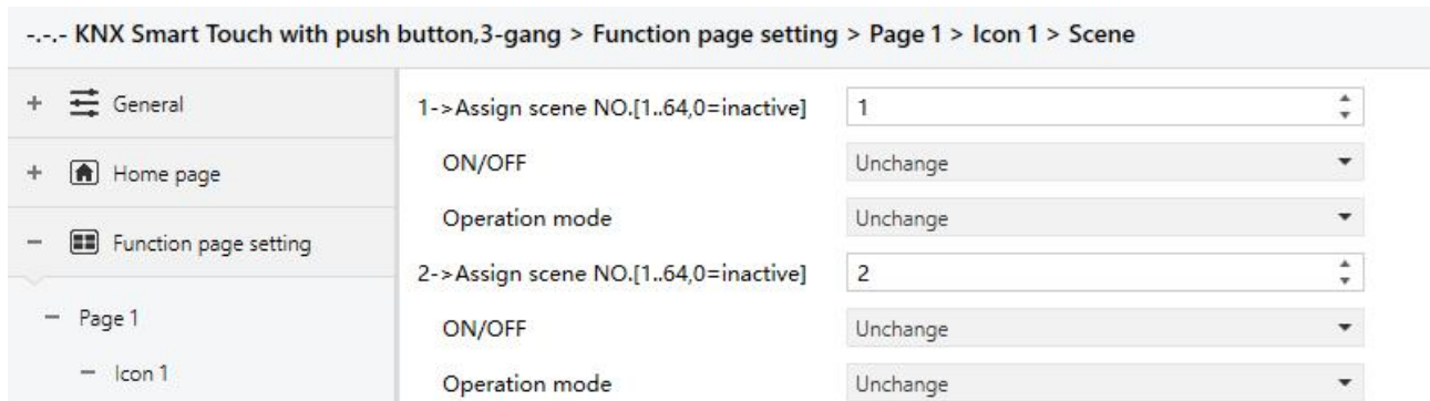
图 5.6.2.3(3) 温控-场景参数设置界面
