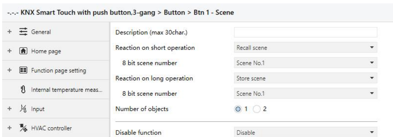
图 5.7.1.4 场景功能参数设置
