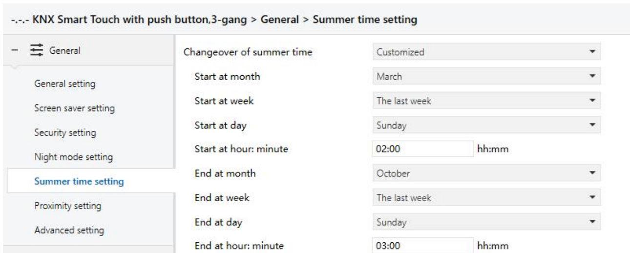
图 5.1.5 “Summer time setting” 参数设置界面
