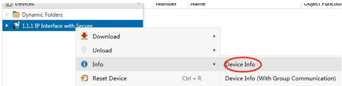
图 4.5 读设备信息
