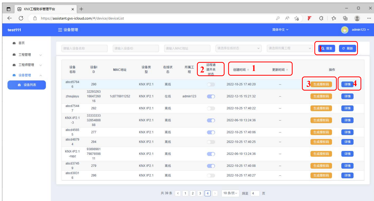
图 7.5.1 设备管理
