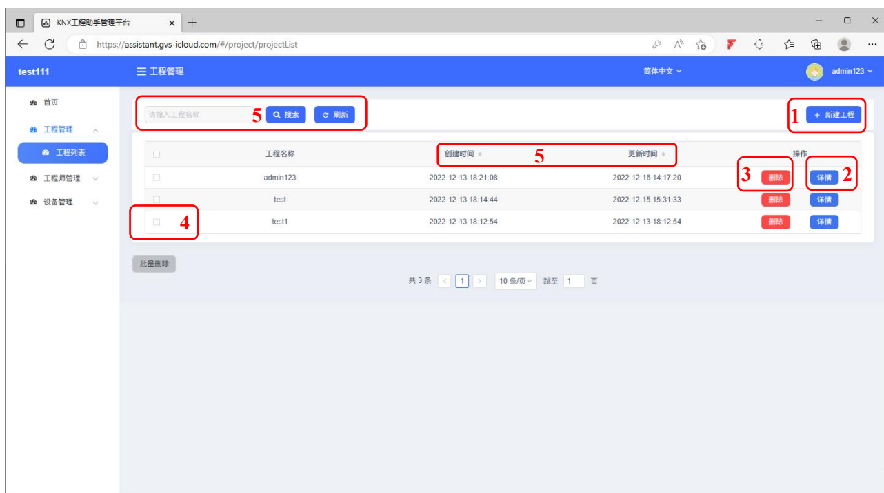
图 7.3.1 工程管理
