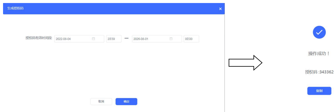
图 7.5.2 生成授权码
