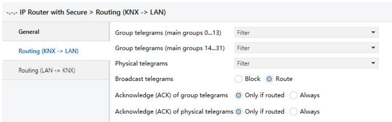
图 5.2 “Routing(KNX->LAN)”参数设置界面
