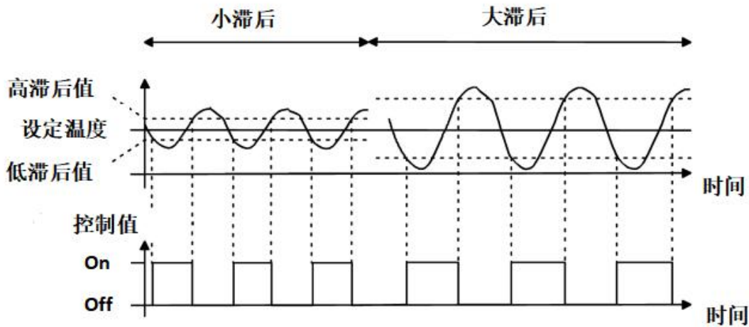
图 5.5.2(2) 两点控制方式下滞后对控制值开关动作的影响 (加热)
