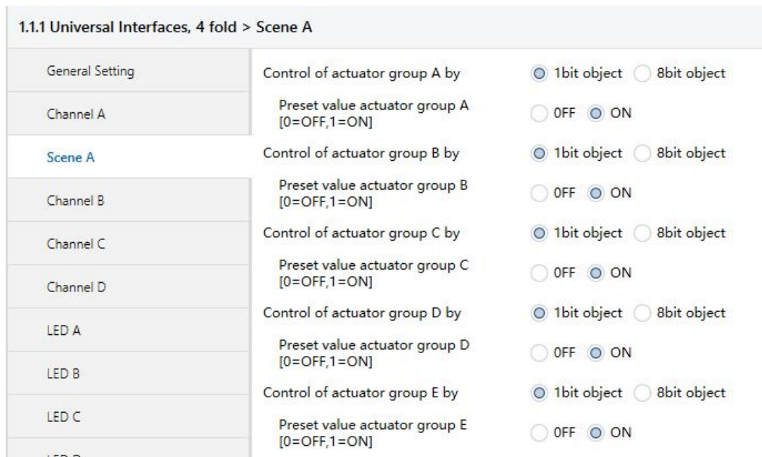
图 10 “scene X”参数设置界面
