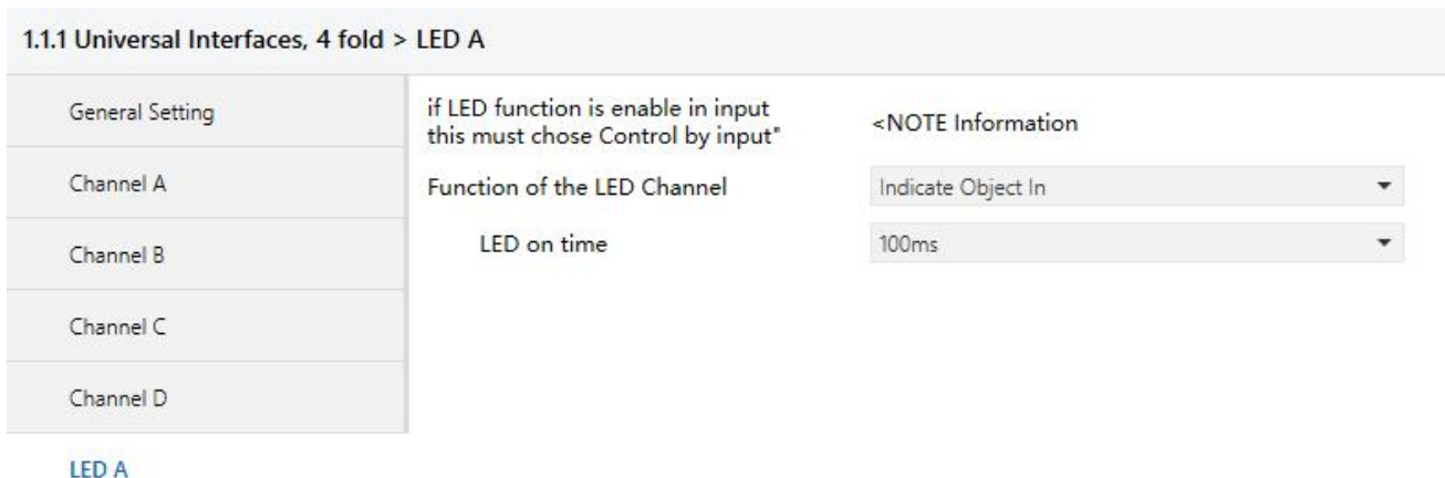
图 19 “Indicate object in, X”参数设置界面
